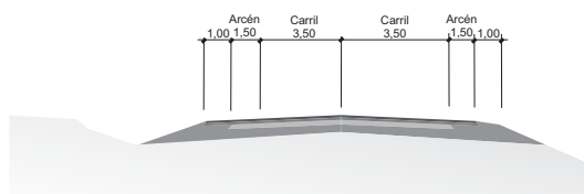
SECCI3N TIPO TRAMO 2
