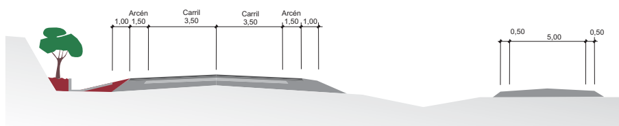
SECCI3N TIPO TRAMO 2
